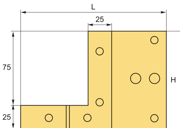
Вид спереди
