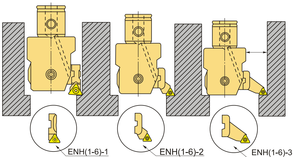
Виды насадок (держатели пластин).
