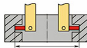
Измерение внутреннего диаметра канавки
