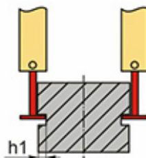
Измерение наружного диаметра канавки ( h1 \leq 3.5 мм)
