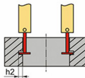
Измерение внутреннего диаметра канавки ( h2 \leq 3.5 мм)
