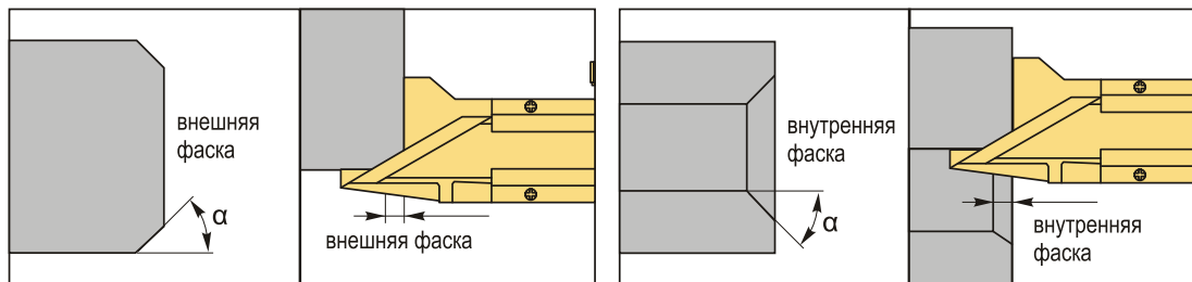
Измерение размера фаски
