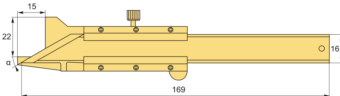
Измерение размера фаски
