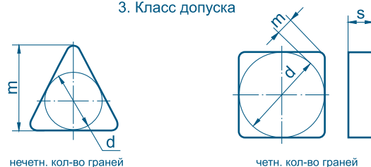
Предельные отклонения размеров, мм
